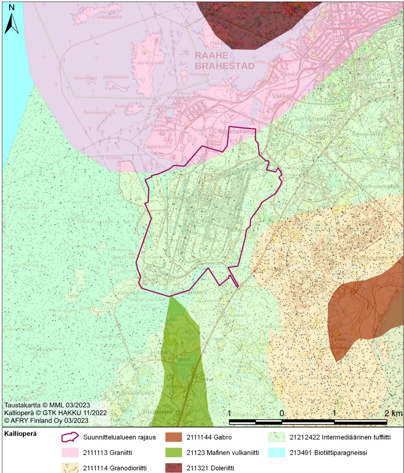
Kuva 4-10. Suunnittelualueen ja sen läheisyyden kallioperä.
