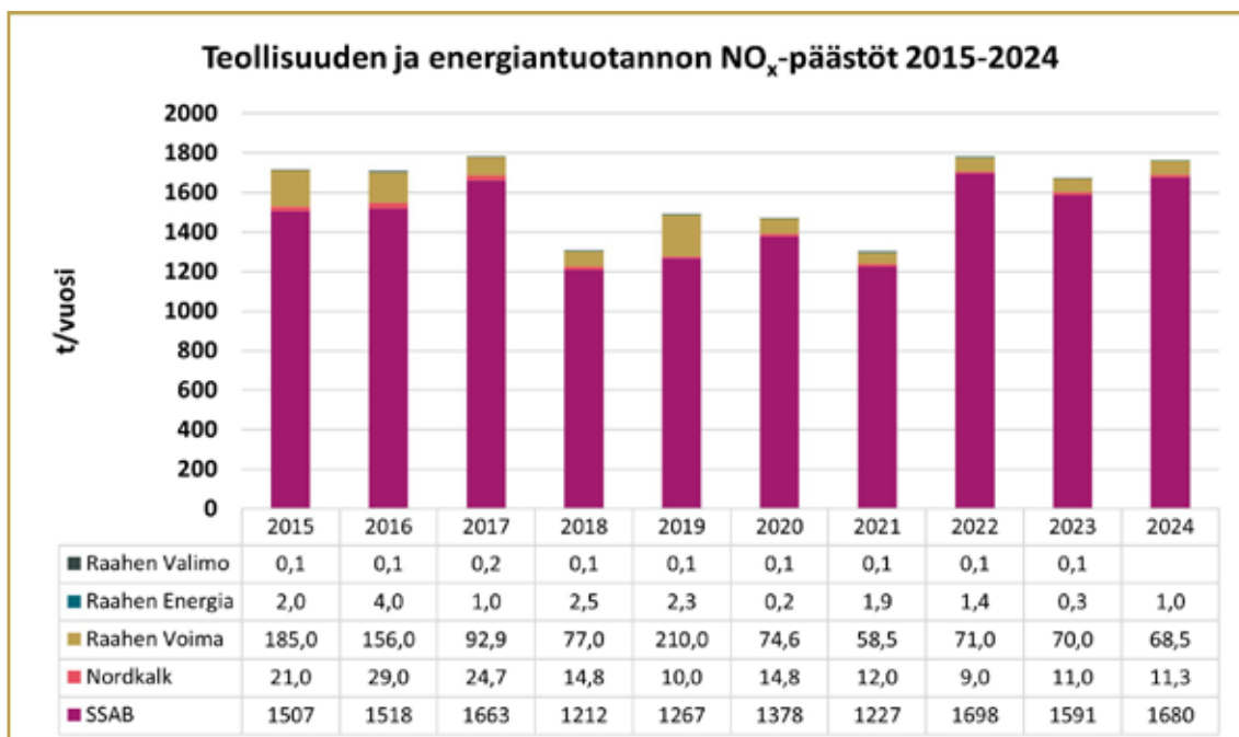
Kaavio 1: Teollisuuden ja energiantuotannon tyyppien oksidipäästöt 2015–2024.
