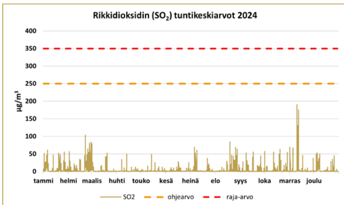
Kaavio 13: Rikkidioksidin tuntikeskiarvot Lapaluodossa sekä ilmanlaatuasetuksen mukaiset tuntikeskiarvon ohjearvo (250 \mu\text{g}/\text{m}^3 ) ja raja-arvo (350 \mu\text{g}/\text{m}^3 ).
