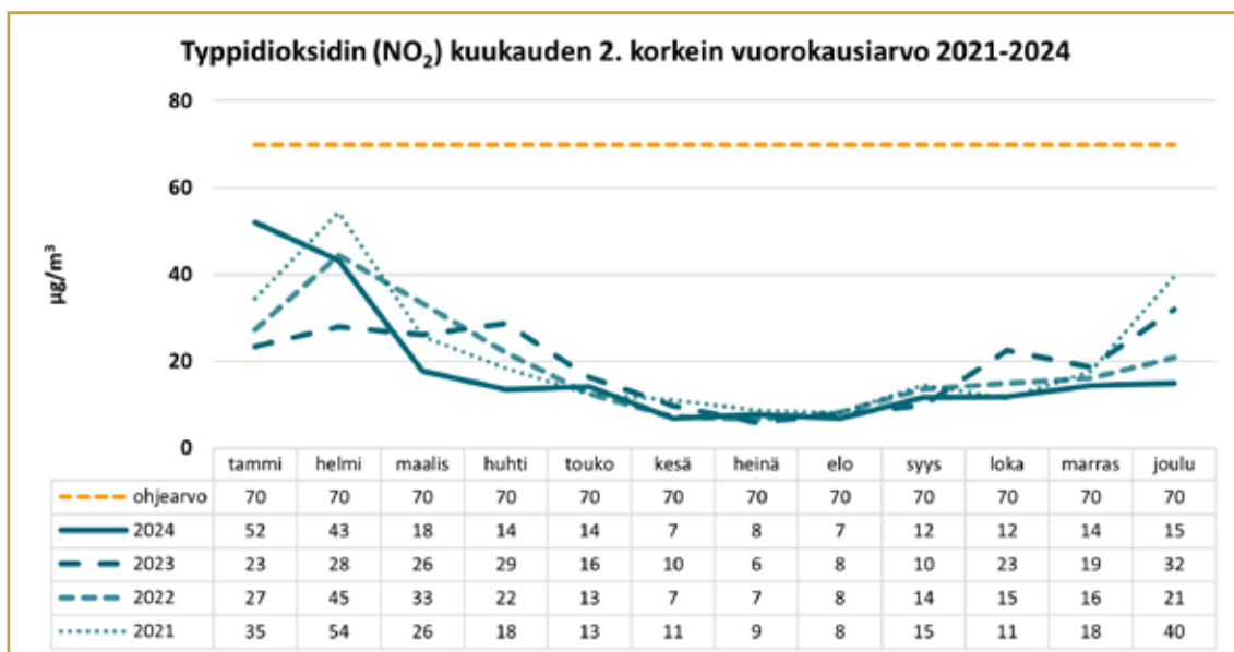
Kaavio 11: Typpidioksidin vuorokausiohjearvoon verrannolliset pitoisuudet kuukausittain vuosina 2021-2024 Keskustassa. Kaavioon on merkitty myös ilmanlaatuasetuksen ohjearvo (70 µg/m 3 ).
