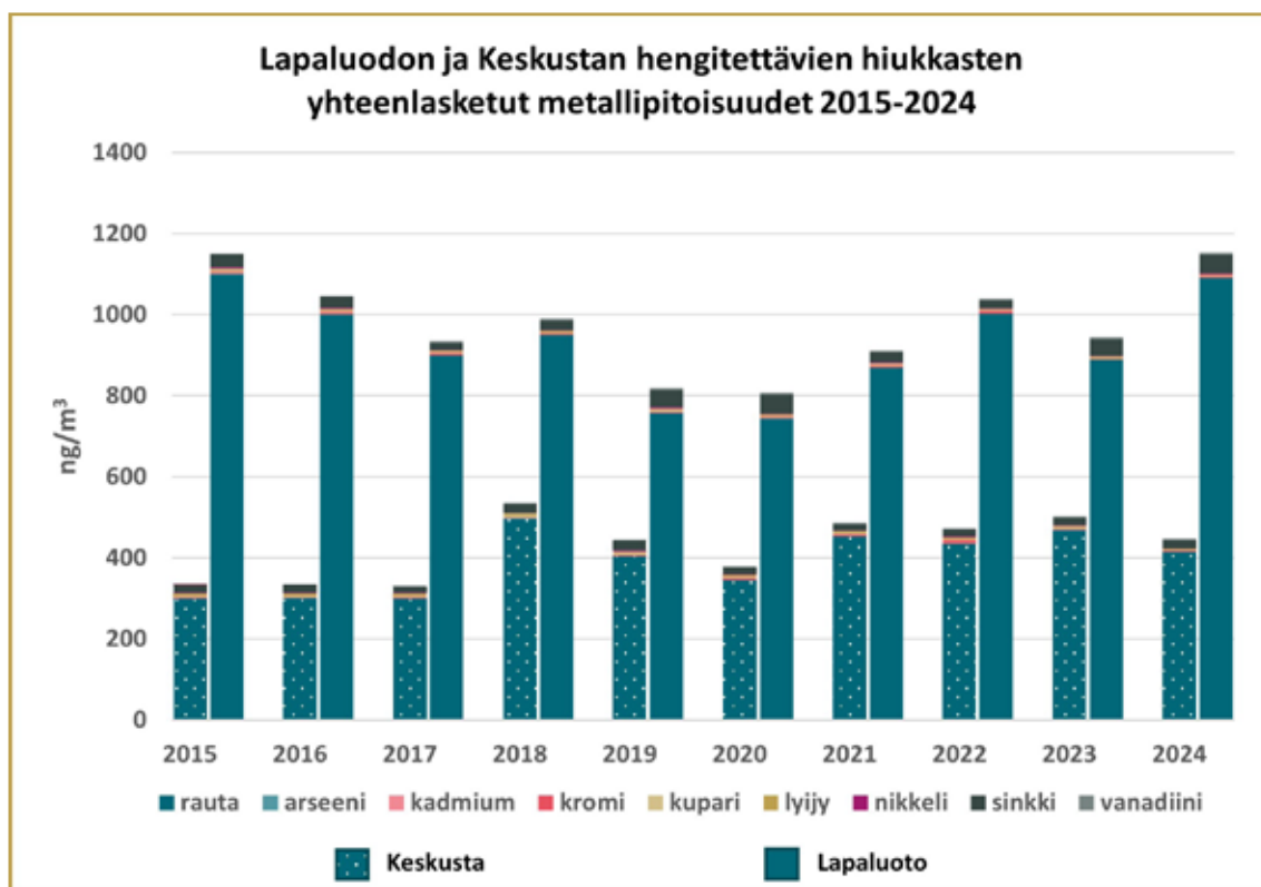
Kaavio 28: Lapaluodon ja Keskustassa mitattujen metallipitoisuuksien yhteenlasketut tulokset 2015–2024.
