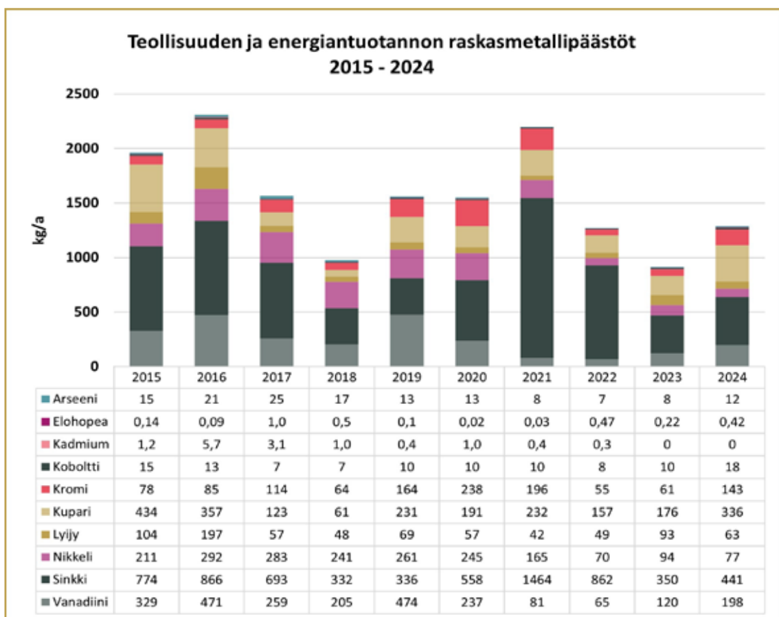
Kaavio 4: Teollisuuden ja energiantuotannon yhteenlasketut raskasmetallipäästöt 2015–2024 ilman rautaa.
