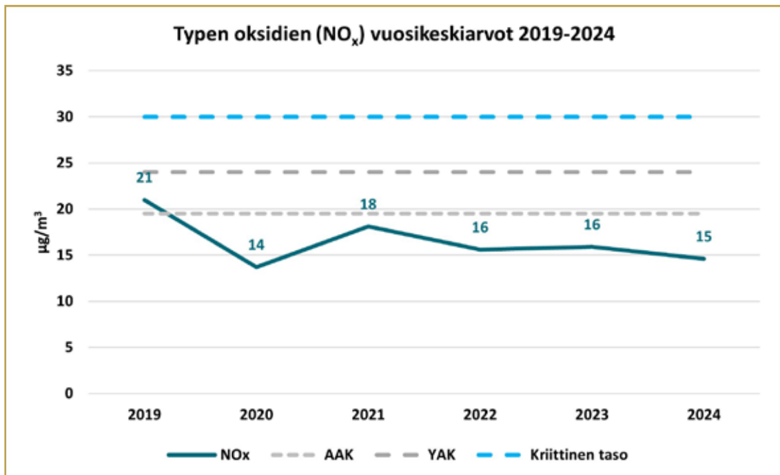
Kaavio 12: Typen oksidien ( \text{NO}_x ) vuosikeskiarvot Keskustassa. Kaavioon on merkitty myös kriittinen taso ( 30 \mu\text{g}/\text{m}^3 ), alempi arviointikynnys ( 19,5 \mu\text{g}/\text{m}^3 ) ja ylempi arviointikynnys ( 24 \mu\text{g}/\text{m}^3 ).
