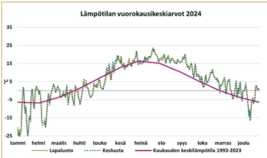
Kaavio 40: Lapuudon ja Keskustan lämpötilan vuorokausikeskiarvot sekä pitkän ajan kuukausikeskiarvo. Lapuudon säätiedot ovat Ilmatieteen laitoksen sääasemalta.
