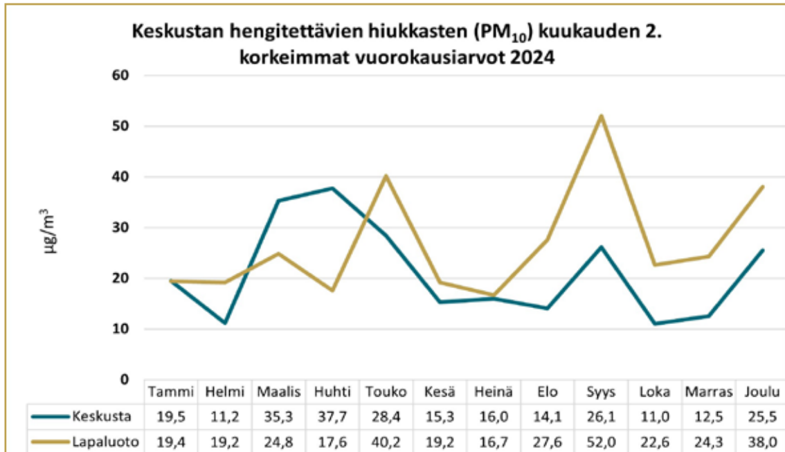
Kaavio 22: Hengitettävien hiukkasten ( \text{PM}_{10} ) kuukauden 2. suurimmat vuorokausiarvot kuukausittain Keskustan mitausasemalla.
