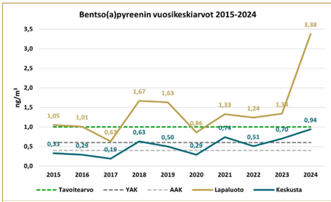
Kaavio 25: Bentso(a)pyreenin vuosikeskiarvo 2015–2024. Käyrien päällä oleva lukuarvo kuvaa kunkin vuoden mitattua vuosikeskiarvoa. YAK = Ylempi arviointikynnys ( 0,6 \text{ ng/m}^3 ) ja AAK = alempi arviointikynnys ( 0,4 \text{ ng/m}^3 ).
