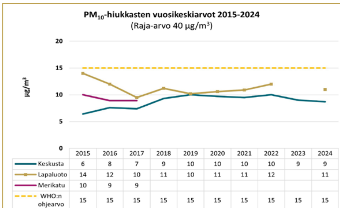
Kaavio 19: Hengitettävien hiukkasten vuosikeskiarvot 2015–2024. Kaavioon on merkitty lisäksi WHO:n ohjearvo. Vuosikeskiarvon raja-arvo on 40\text{ }\mu\text{g}/\text{m}^3 .
