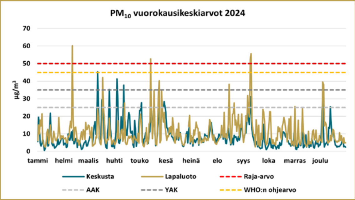
Kaavio 21: PM 10 vuorokausikeskiarvot. Vuoden aikana sattui yhteensä neljä raja-arvon ( 50 \mu\text{g}/\text{m}^3 ) ylitystä Keskustassa. Kaavioon on merkattu raja-arvon lisäksi ylempi (YAK, 35 \mu\text{g}/\text{m}^3 ) ja alempi (AAK, 25 \mu\text{g}/\text{m}^3 ) arviointikynnys sekä WHO:n ohjearvo ( 45 \mu\text{g}/\text{m}^3 ).
