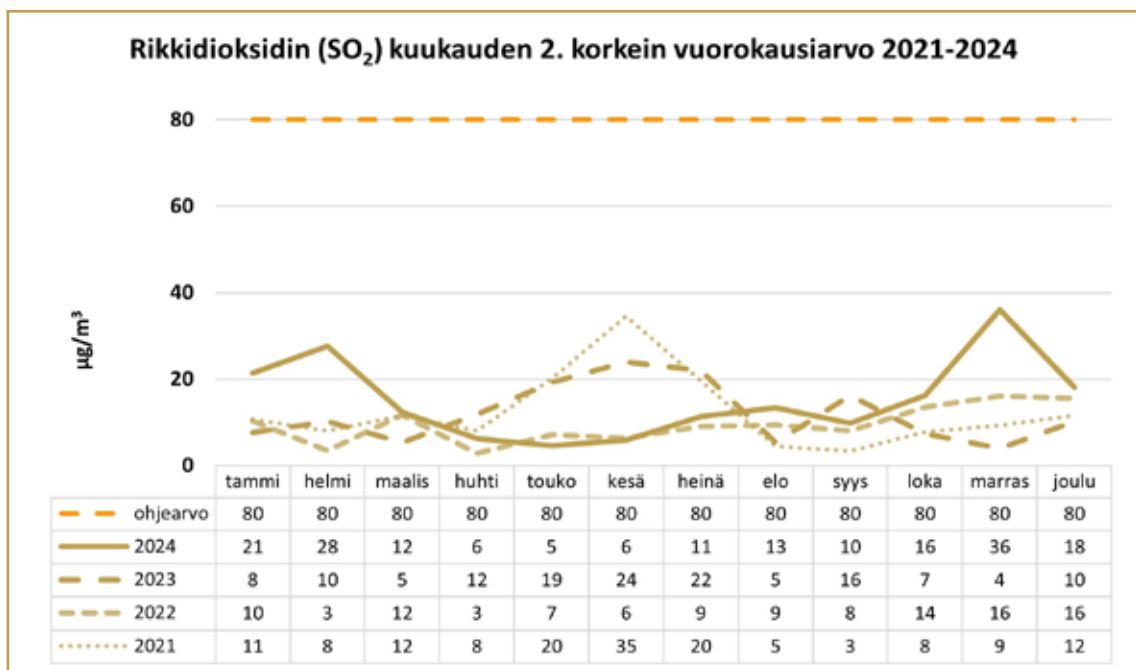
Kaavio 18: Rikkidioksidin vuorokausiohjeeseen verrannolliset pitoisuudet kuukausittain 2021-2024 Lapaluodossa. Kaavioon on merkitty myös ilmanlaatuasetuksen ohjearvo (80 µg/m³).
