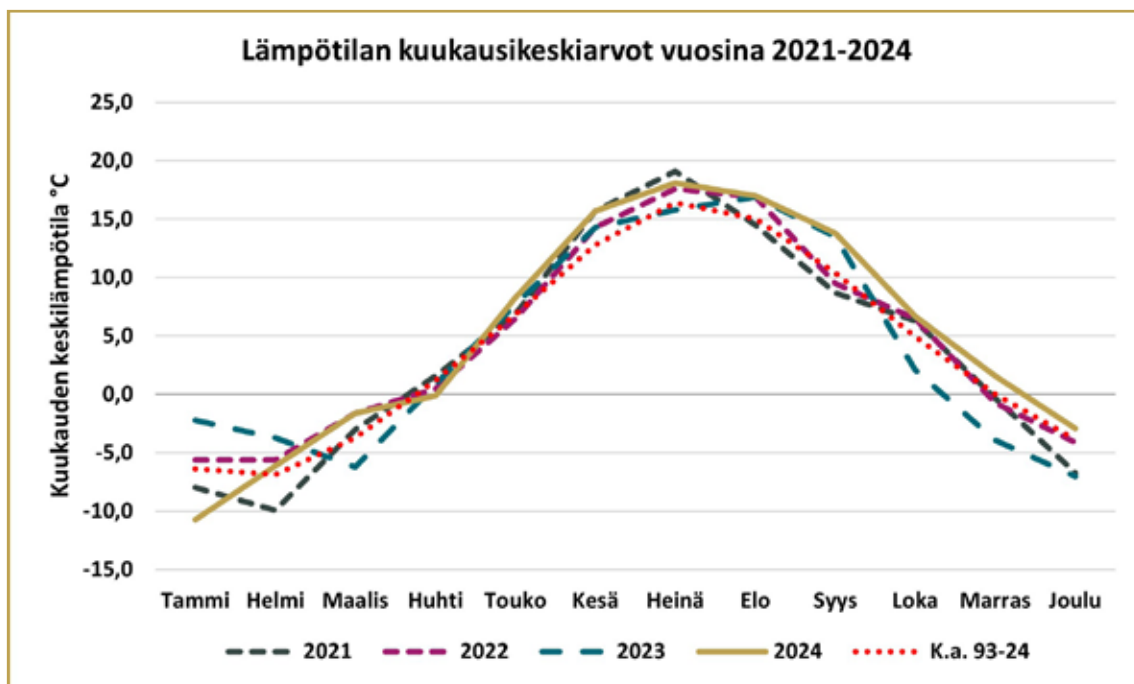
Kaavio 42: Lämpötilan kuukausikeskiarvot vuosina 2021–2024, sekä pitkän ajan kuukausikeskiarvo 1993–2024. Sääti- dot ovat Ilmatieteenlaitoksen Lapaluodon sääasemalta.
