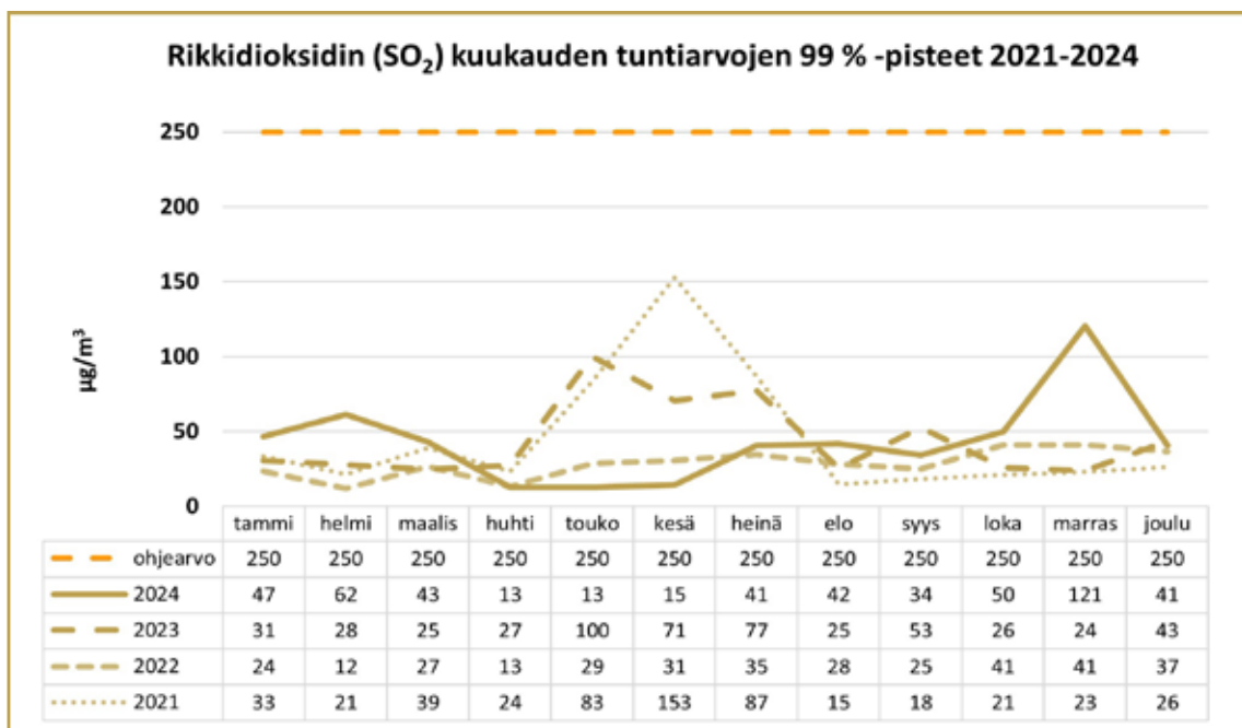
Kaavio 17: Rikkidioksidin tuntiarvoon verrannolliset pitoisuudet 2021-2024 kuukausittain Lapaluodossa. Kaavioon on merkitty myös ilmanlaatuasetuksen ohjearvo (250 µg/m 3 ).
