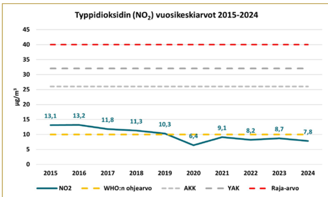
Kaavio 9: Typpidioksidin (NO 2 ) vuosikeskiarvot Keskustassa. Kaavioon on merkitty myös vuosikeskiarvon raja-arvo (40 µg/m³), alempi arviointikynnys (26 µg/m³), ylempi arviointikynnys (32 µg/m³) ja WHO:n ohjearvo (10 µg/m³).
