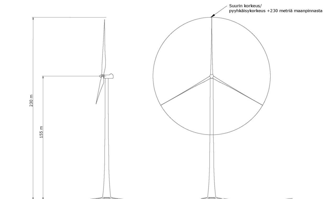
Kuva 2. 230 metriä korkea tuulivoimala.
