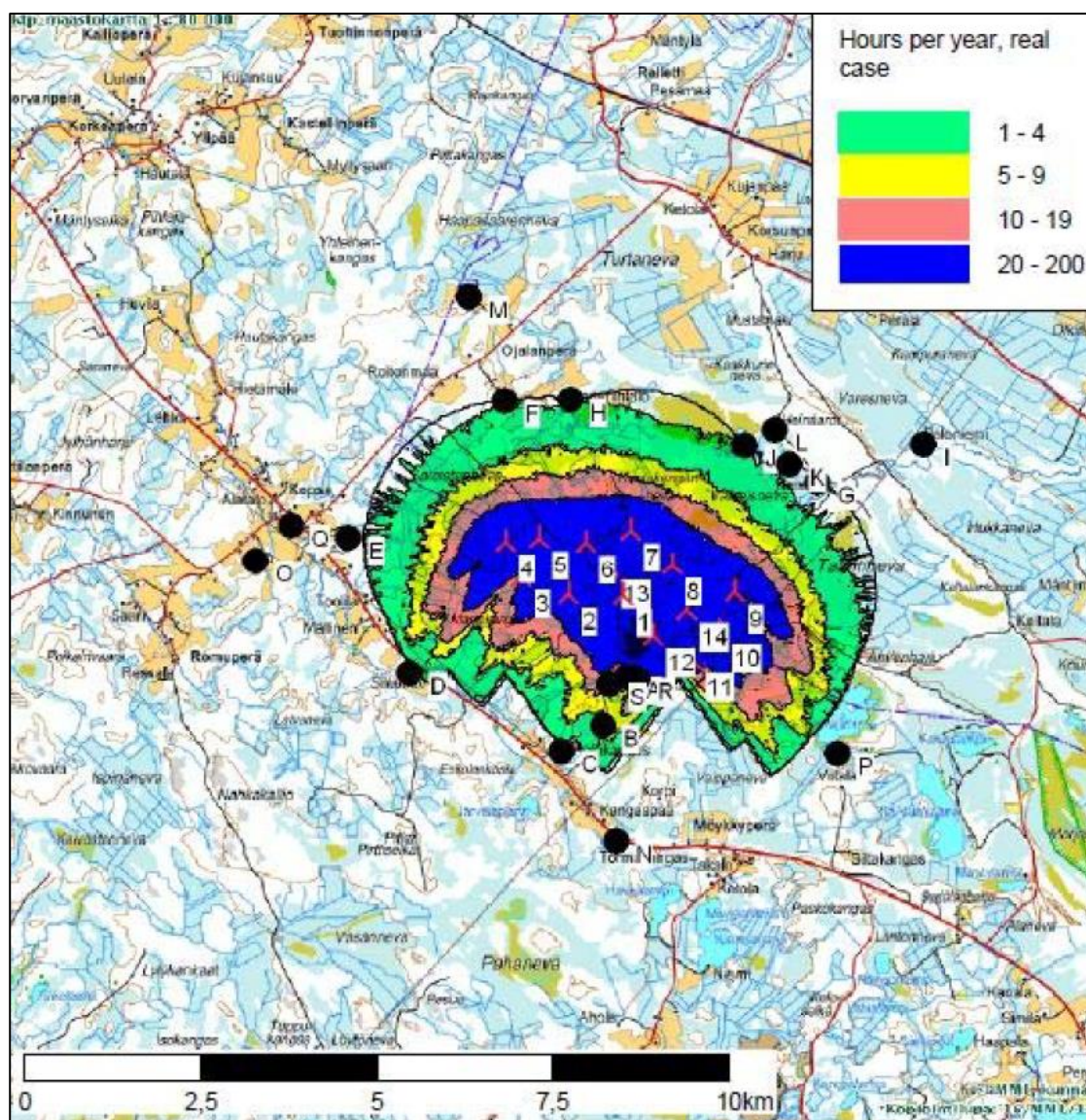
Kuva 19. Kaavaselostuksen Kuva 2.9. Mastokankaan tuulivoimapuiston välkevaikutusten vyöhykkeet. Kirjaimet A–S viittaavat tarkkailupisteisiin.
