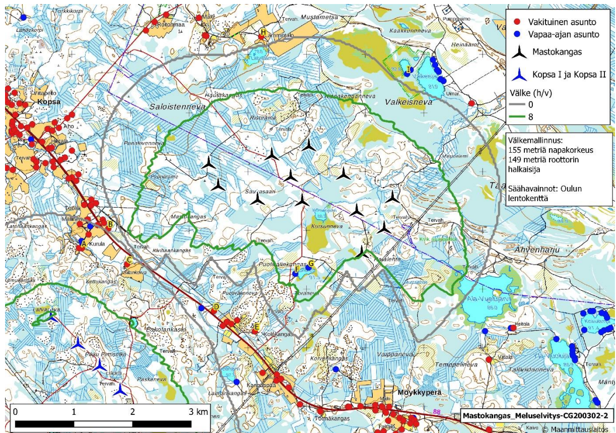
Kuva 2. Varjovälkkeen muodostuminen Mastokankaan alueella. Havainnointipisteet on merkitty kuvaan (a-k) ja niiden välketasot on esitetty taulukossa 5.
