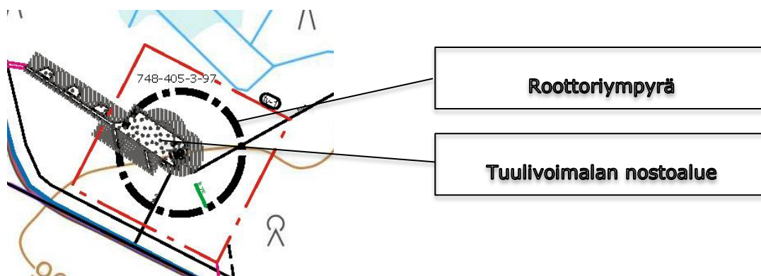
Kuva 1. Tuulivoimalan nostoalue tv-alueella.
