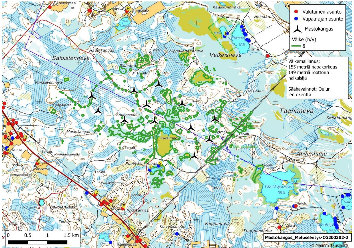
Kuva 6. Varjovälkkeen muodostuminen Mastokankaan alueella puuston suojaava vaikutus huomioiden. Havainnointipisteet on merkitty kuvaan (A-I) ja niiden vältketasot on esitetty taulukossa 6.
