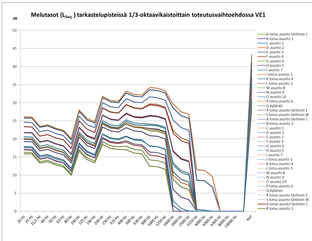
Kuva 7-4. Mastokankaan tuulivoimapuiston aiheuttamat melutasot taajuuskaistoittain vaihtoehdossa VE1.
