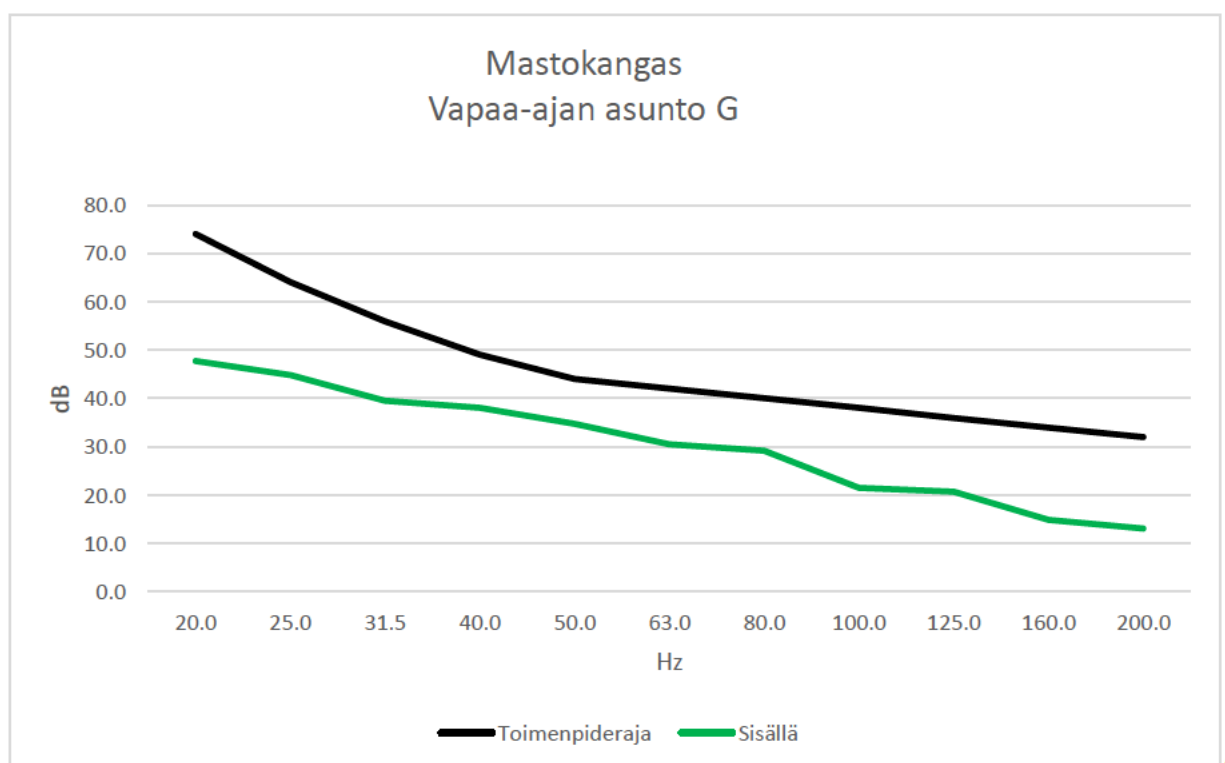
Kuva 5. Ympäristöministeriön ohjeistuksen mukainen pienitaajuisen melun laskenta sekä sosi-aali- ja terveysministeriön toimenpiderajat vapaa-ajan asunnossa G.
