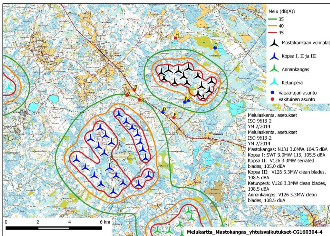
Kuva 15. Kaavaselostuksen Kuva 2.7. Mastokankaan tuulivoimapuiston yhteisvaikutusten melumallinnus 6.3.2016. Kuvaan on merkitty havainnointipisteet.
