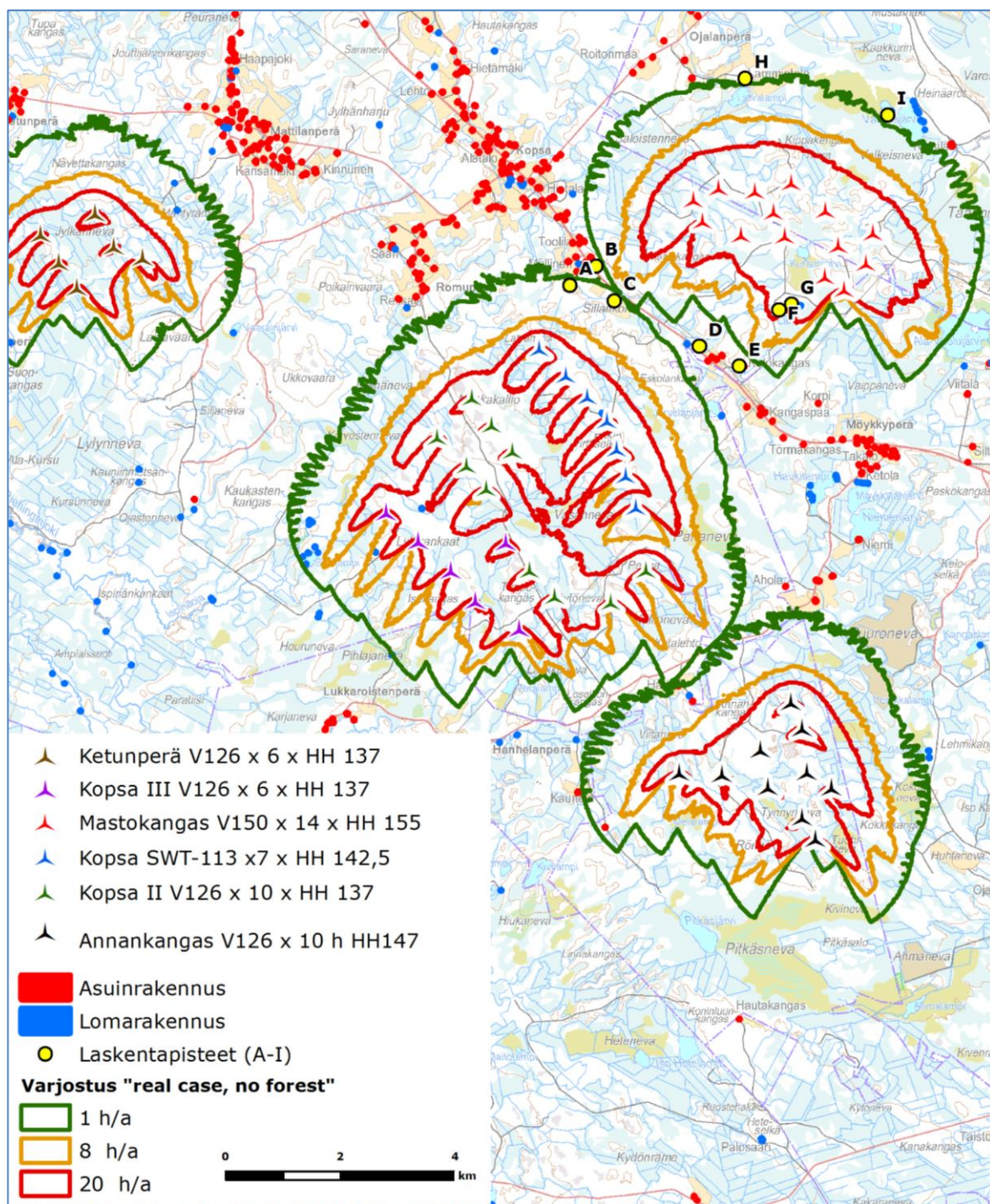
Kuva 20. Mastokankaan hankkeen laskennalliset varjostustulokset, kun huomioidaan jo tuotannossa olevat voimalat ja lähiseudun suunnitteilla olevat tuulivoimahankkeet. Yhteensä 53 tuulivoimalaa. Laskelmissa suojaavaa puustoa EI ole huomioitu.
