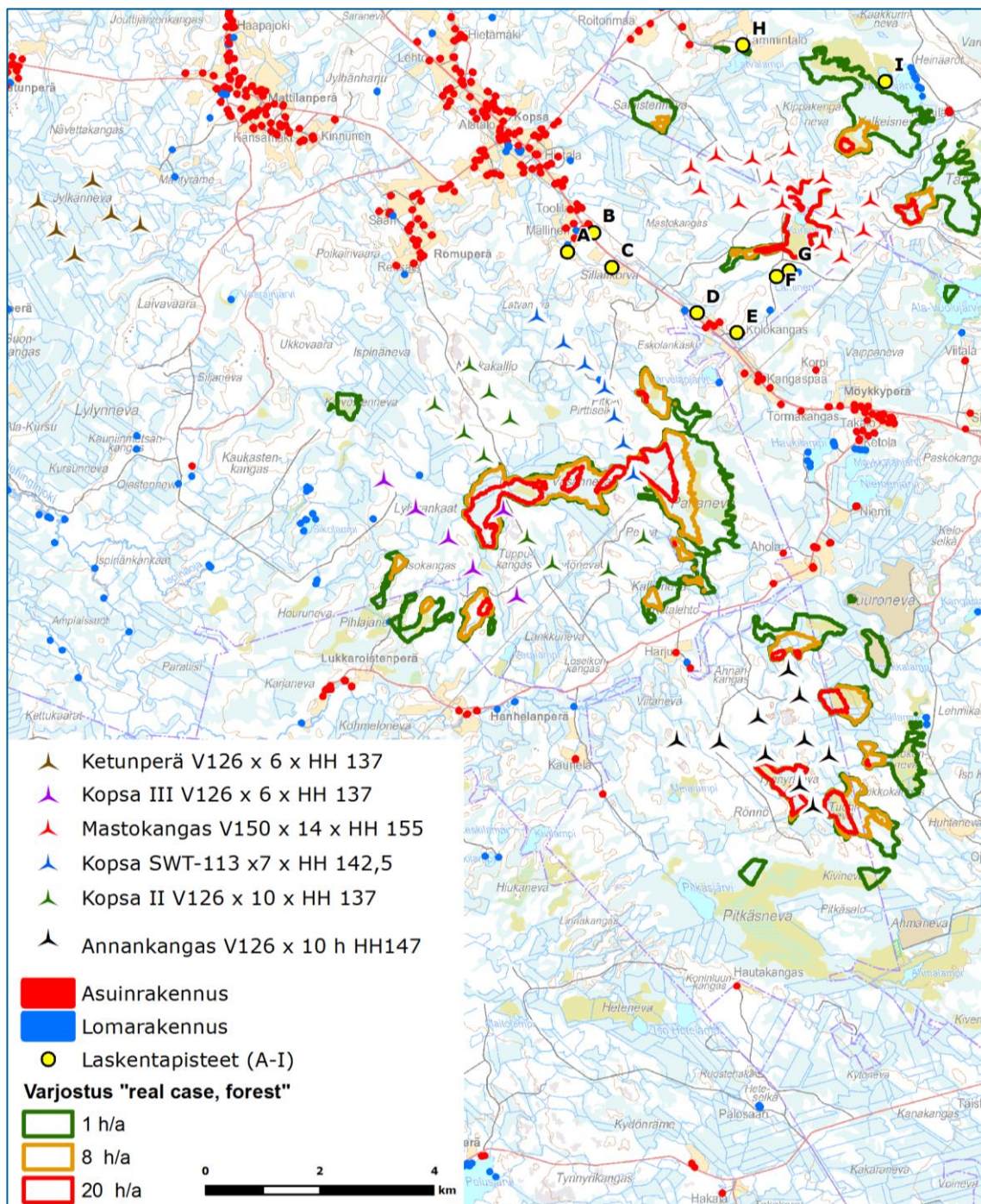
Kuva 21. Mastokankaan tuulivoimapuiston laskennalliset varjostustulokset, kun huomioidaan tuotannossa olevat voimalat ja lähiseudun suunnitteilla olevat tuulivoimahankkeet, yhteensä 53 tuulivoimalaa. Laskelmissa suojaava puusto on huomioitu.
