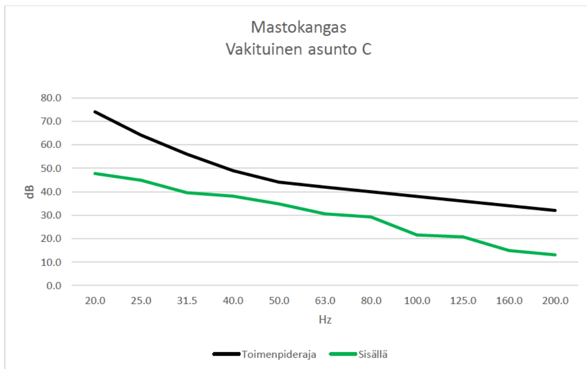
Kuva 4. Ympäristöministeriön ohjeistuksen mukainen pienitaajuisen melun laskenta sekä sosi-aali- ja terveysministeriön toimenpiderajat vakituksessa asunnossa C.
