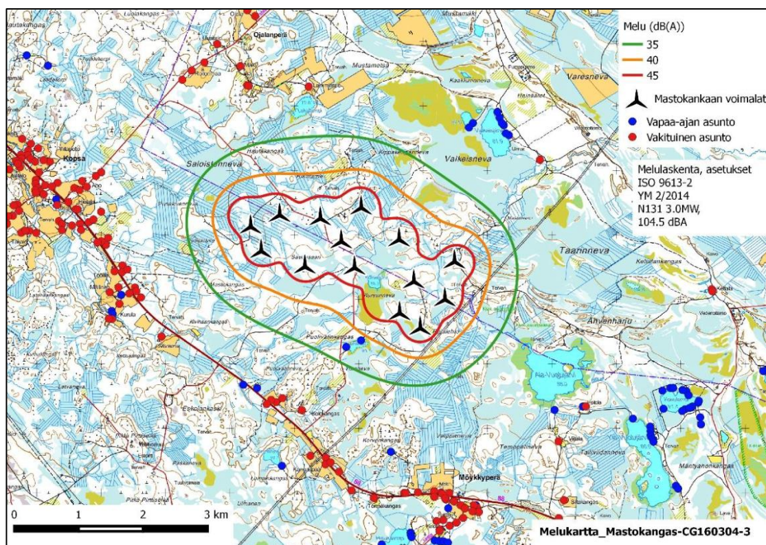
Kuva 14. Kaavaselostuksen Kuva 2.6. Mastokankaan tuulivoimapuiston melumallinnus 6.3.2016.
