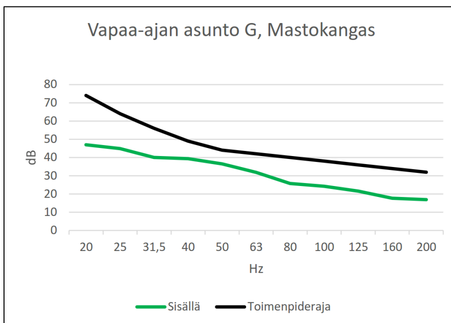
Kuva 17. Kaavaselostuksen Kuva 2.8. Ympäristöministeriön ohjeistuksen mukainen pienitaajuisen melun laskenta sekä sosiaali- ja terveysministeriön toimenpiderajat vapaa-ajan asunnossa G.
