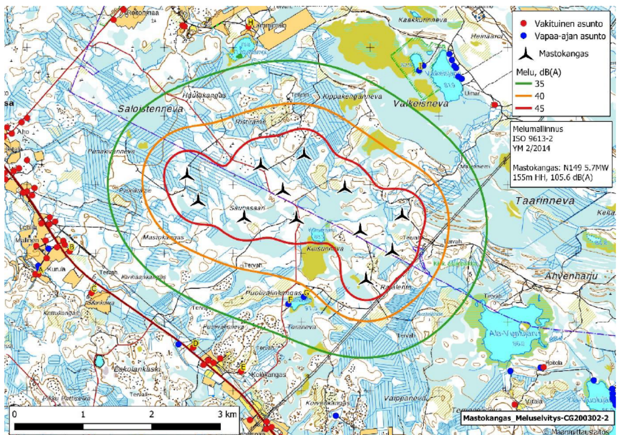
Kuva 6-1. Mastokankaan tuulivoimapuiston melumallinnus, N149 5.7 MW 105,6 dB(A). Kuvassa 9 havainnointipistettä on merkitty kirjaimilla.
