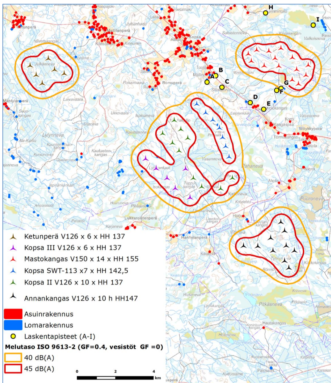
Kuva 16. Mastokankaan, lähialueen rakennettujen tuulivoimapuistojen ja suunnitteilla olevien tuulivoimahankkeiden laskennalliset yhteismelutasot. Yhteensä 53 tuulivoimalaa. Mallinnus 30.7.2018. Kuvaan on merkitty havainnointipisteet.
