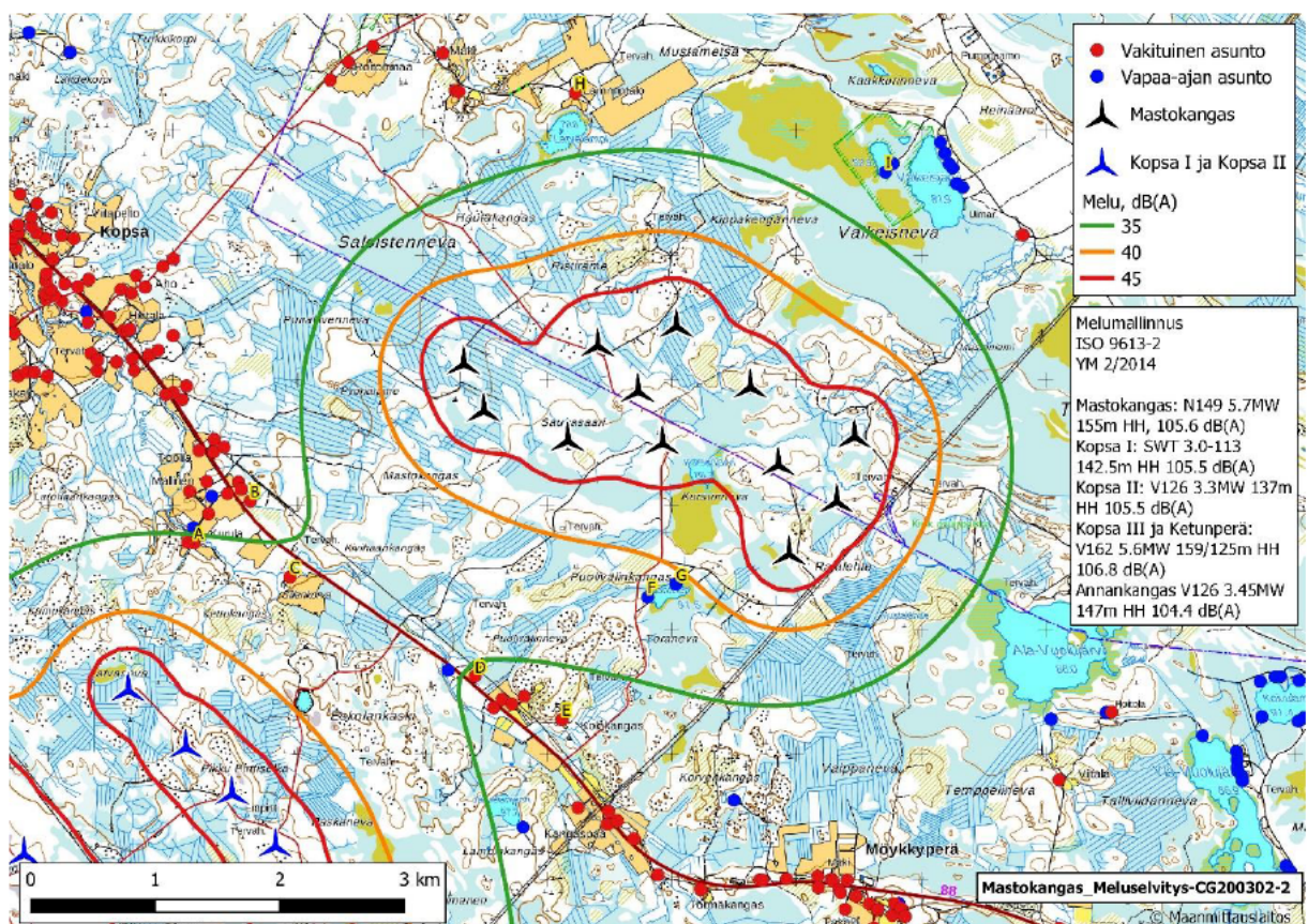
Kuva 6-2. Mastokankaan tuulivoimapuiston melumallinnus, N149 5.7 MW 105,6 dB(A). Kuvassa 9 havainnointipistettä on merkitty kirjaimilla.
